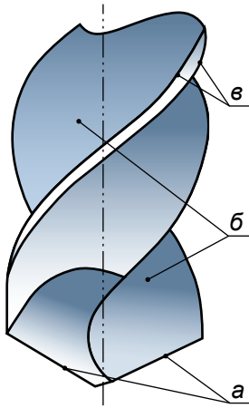
Мал. 73. Конструкція робочої частини свердла: а – різальні кромки; б – гвинтові канавки; в – спіральні стрічки
