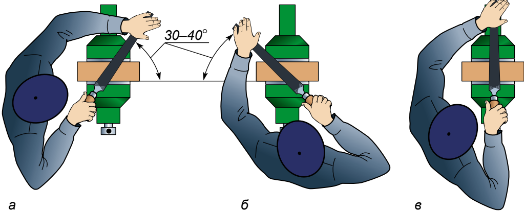
Мал. 98. Способи обпилювання: а – зліва направо; б – справа наліво; в – прямо
