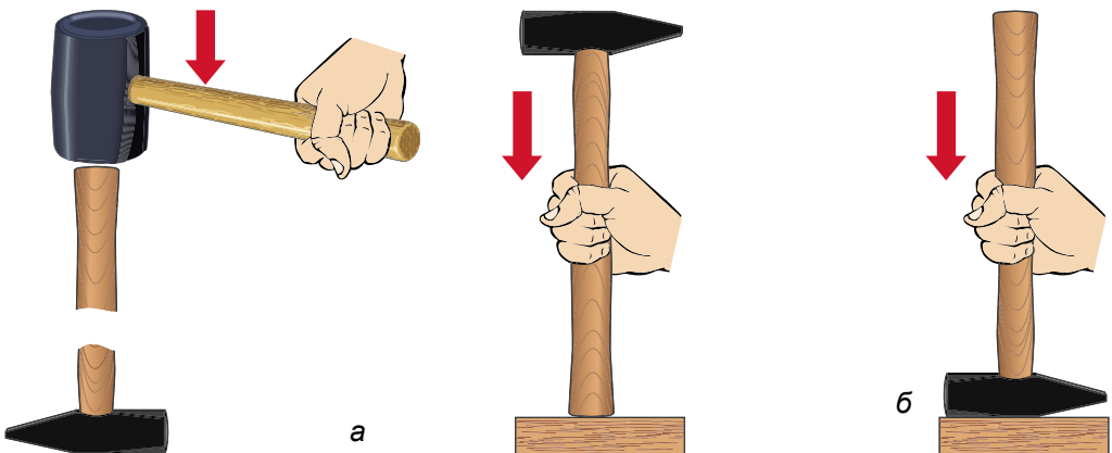
Мал. 119. Насадження бойка молотка: а – правильне; б – неправильне
