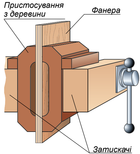
Мал. 94. Кріплення заготовки в пристосуванні
