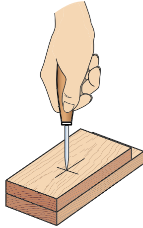
Мал. 115. Наколювання місць заби- вання
