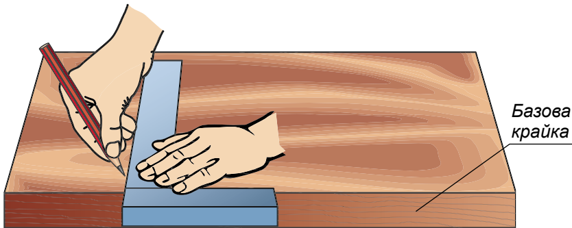
Мал. 42. Розмічання кутником від базової крайки
