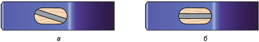
Мал. 118. Схеми кріплення бойка молотка за допомогою клина: а – правильно; б – неправильно
