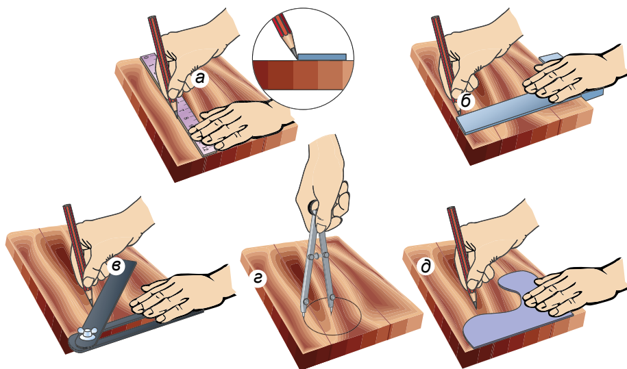
Мал. 43. Прийоми розмічання: а – лінійкою; б – кутником; в – малкою; е – циркулем; д – шаблоном
