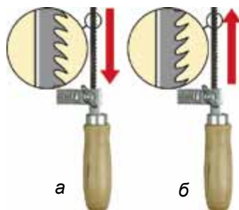
Мал. 55. Кріплення пилочки в рамці: а – правильне; б – неправильне
