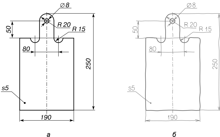
Мал. 36. Графічні зображення: а – креслення деталі; б – ескіз
