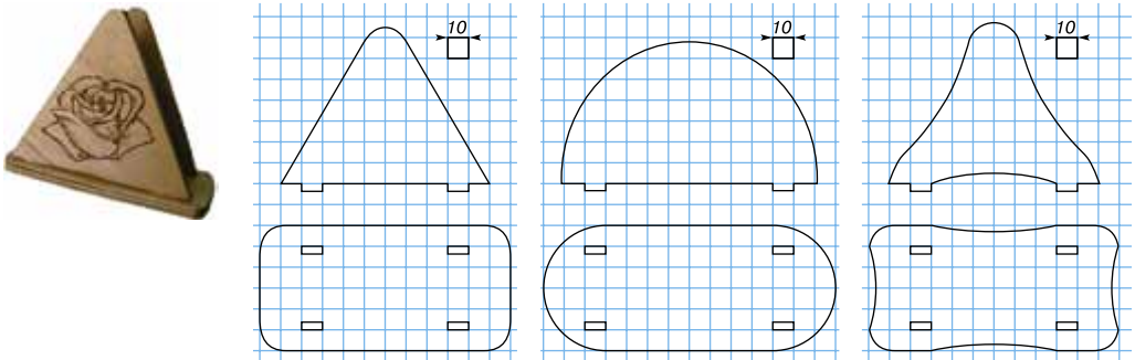
Мал. 67. Варіанти контурів серветниць
