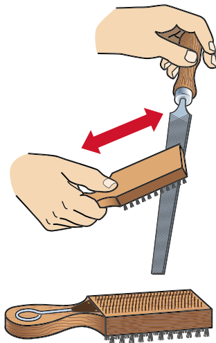
Мал. 100. Очищення напилка металевою щіткою
