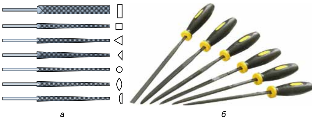
Мал. 92. Види надфілів: а – схематичне зображення; б – загальний вигляд
