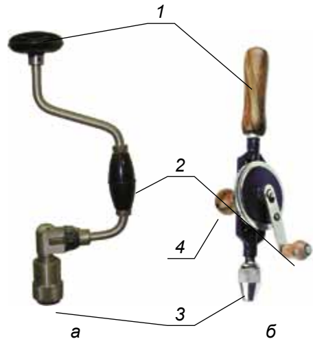
Мал. 75. Ручні свердлильні інструменти: а – коловорот; б – ручний дріль. 1 – упорна ручка; 2 – ручка для обертання; 3 – патрон; 4 – ручка допоміжна
