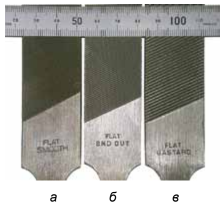
Мал. 90. Види напилків: а – бархатний; б – личкувальний; в – драчевий
